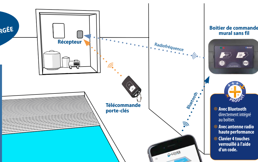
Exemple d'installation avec une mécanique immergée
