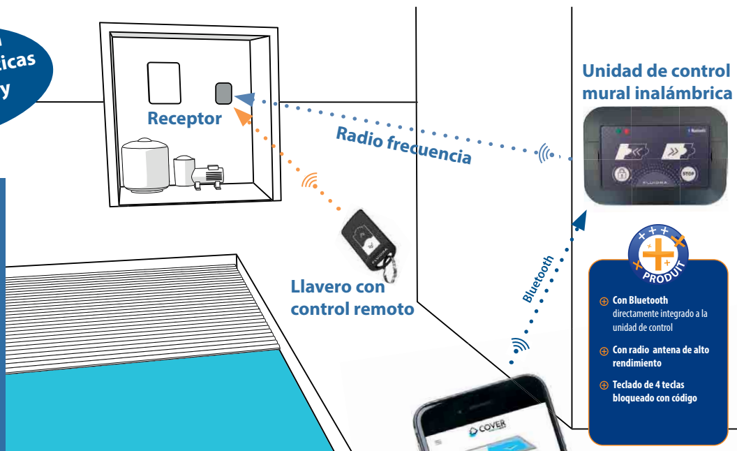
Ejemplo de instalación de una unidad sumergida
